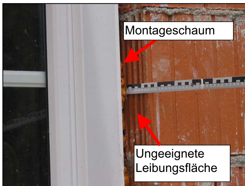
Abbildung 3 : In der Praxis häufig vorzufindende mangelhafte Fugenausbildung.
